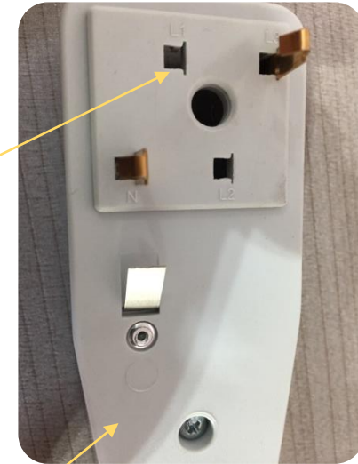
Ranuras marcadas para seleccionar los conductores
