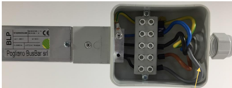
Caja de alimentación, para energizar electroducto de alumbrado.
